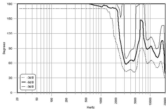
Beamwidth
